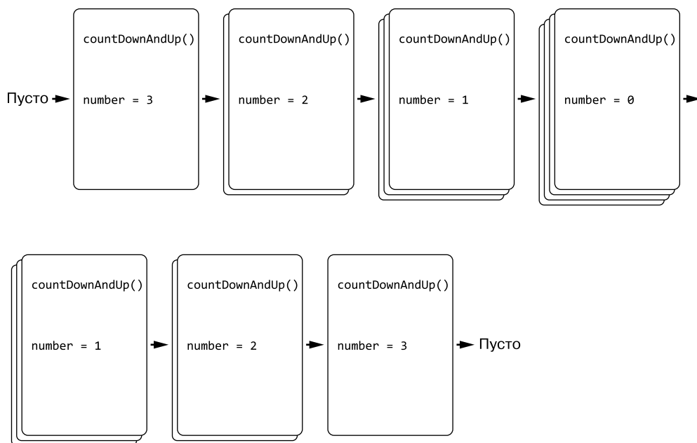
Рис. 1.9. Состояние стека вызовов, отслеживающего значения локальной переменной number при каждом вызове функции
