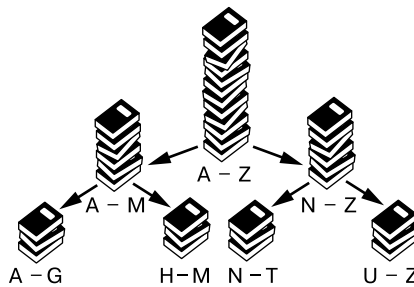
Рис. 5.2. Быстрая сортировка предполагает многократное разбиение коллекции элементов на два набора
