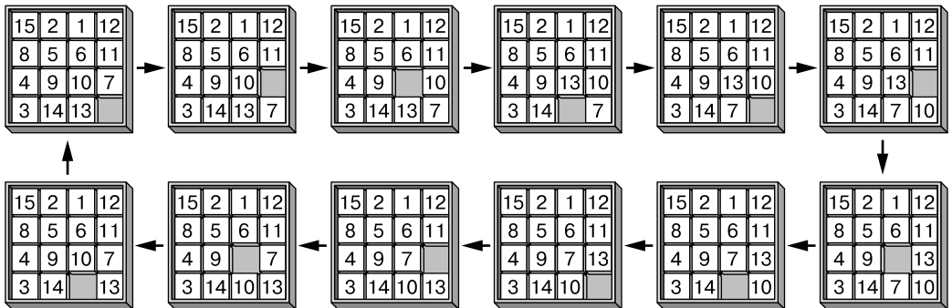
Рис. 12.4. Пример петли в графе алгоритма для решения «пятнашек»
