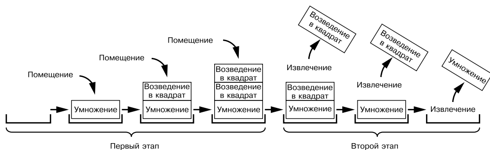
Рис. 2.4. Изменение состояния стека opStack по мере выполнения вызовов функции WithPowerRule(6, 5)
