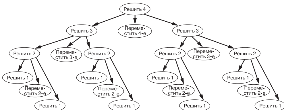
Рис. 3.5. Последовательность операций для решения головоломки «Ханойская башня» из четырех колец
