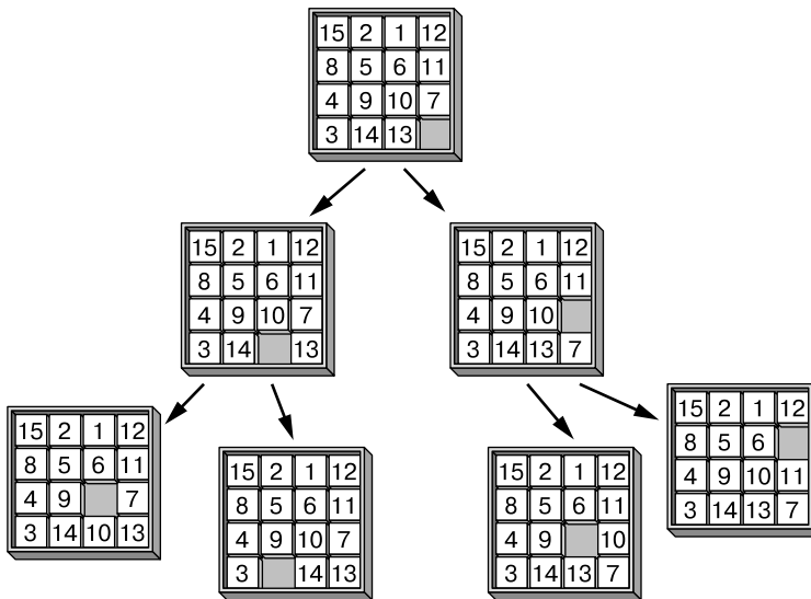
Рис. 12.2. Процесс решения «пятнашек» может быть представлен в виде графа, узлы которого соответствуют состояниям головоломки, а ребра — вариантам перемещения костяшек
