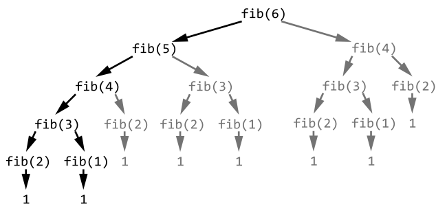
Рис. 7.1. Древовидная диаграмма рекурсивных вызовов функций, начиная с fibonacci(6) . Избыточные вызовы выделены серым цветом
