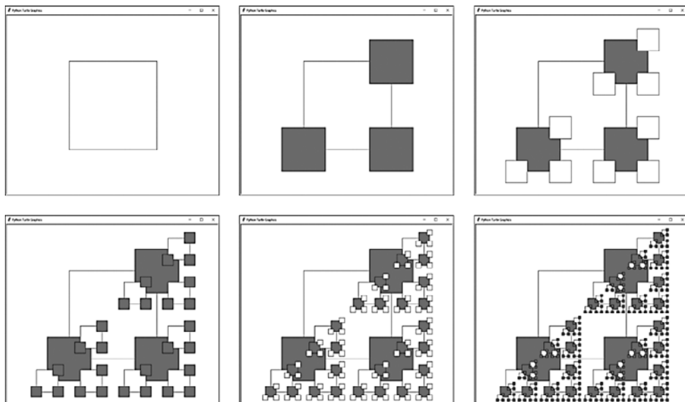
Рис. 13.9. Фрактал «Четыре угла», полученный в результате удаления первого словаря из списка specs
