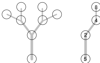
Рис. 3.2. Массив [5, 2, 4, 8] (справа) подобен древовидной структуре данных (слева), имеющей только одну ветвь, выходящую из каждого узла
