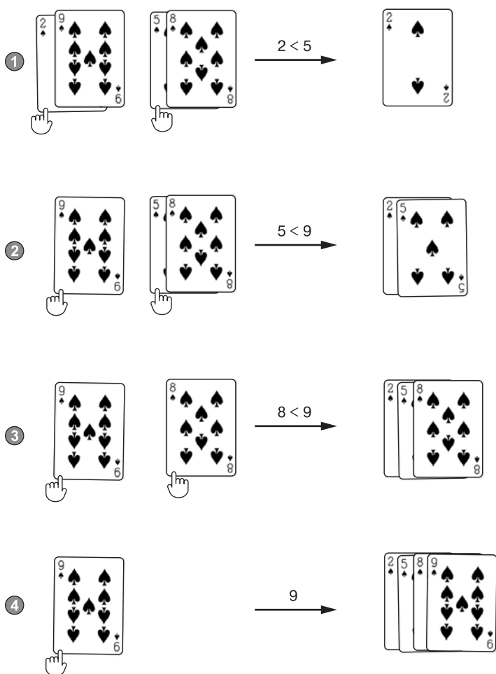
Рис. 5.4. На этапе слияния производится сравнение начальных значений небольших отсортированных списков и добавление меньшего из них в большой список. Для слияния списков, содержащих в общей сложности четыре карты, требуется всего четыре шага
