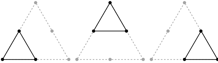
Рис. 9.4. Три внутренних треугольника с вершинами в равноудаленных точках
