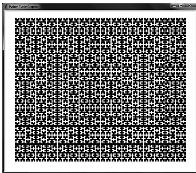
Рис. 9.19. Результат создания заполненной цветом кривой Гильберта при использовании шести уровней рекурсии и линии длиной 5
