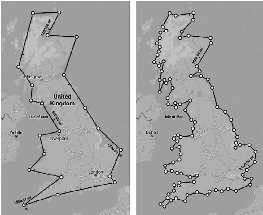
Рис. 9.13. Карта Великобритании с приблизительной длиной береговой линии (слева) и более точной (справа). Во втором случае длина береговой линии больше на 1280 км
