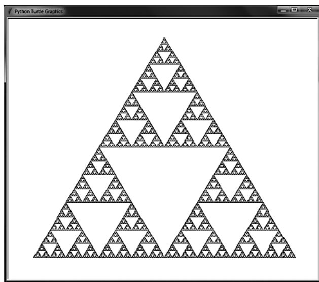
Рис. 9.5. Стандартный треугольник Серпинского
