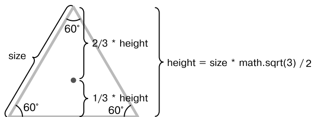
Рис. 13.6. Параметры равностороннего треугольника, длина стороны которого равна значению параметра size
