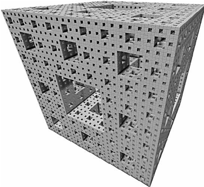
Рис. 9.10. Трехмерный фрактал под названием «губка Менгера»
