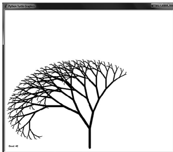
Рис. 9.11. Идеально самоподобное фрактальное дерево, полученное при использовании одинаковых углов и соотношений длин ветвей
