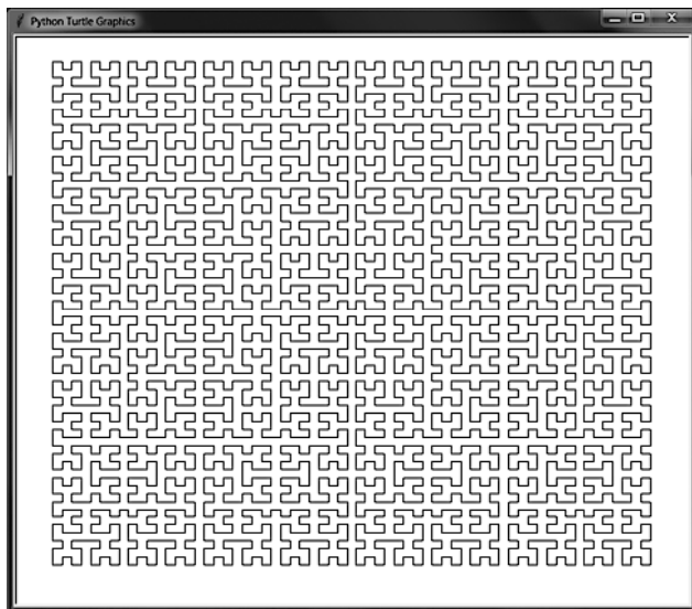
Рис. 9.18. Результат создания кривой Гильберта при использовании пяти уровней рекурсии и линии длиной 10
