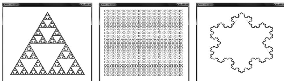
Рис. В.1. Примеры фракталов: треугольник Серпинского (слева), кривая Гильберта (в центре) и снежинка Коха (справа)
