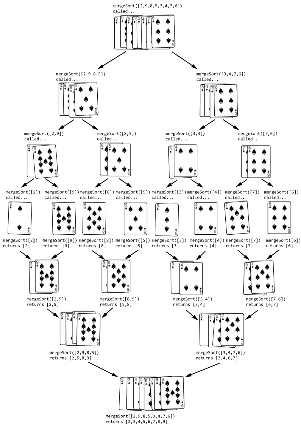
Рис. 5.3. Этапы процесса сортировки слиянием
