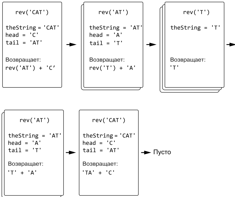
Рис. 3.3. Изменение состояния стека вызовов в процессе обращения строки CAT с помощью функции rev()
