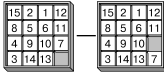
Рис. 12.3. Ребра древовидного графа «пятнашек» не являются направленными (рисуются без стрелки), потому что перемещение костяшки можно отменить, вернув ее в исходное положение
