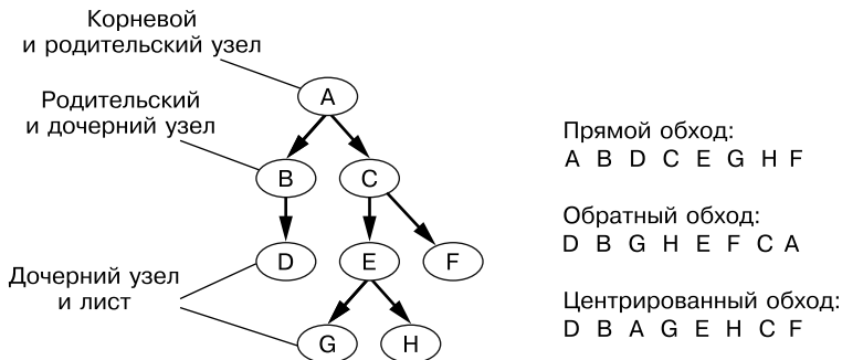
Рис. 4.2. Дерево с корнем A и листьями D, G, H и F, а также способы его обхода
