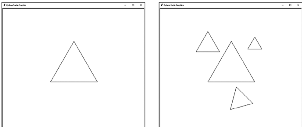
Рис. 13.3. Треугольник, созданный в результате первого вызова drawFractal() (слева), и треугольники, полученные в результате трех рекурсивных вызовов (справа)
