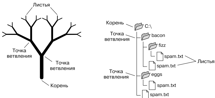
Рис. 2.6. Структура файловой системы напоминает дерево
