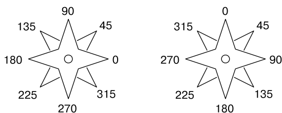
Рис. 9.2. Направления движения черепашки в модуле Python turtle (слева) и в библиотеке JavaScript jtg (справа)
