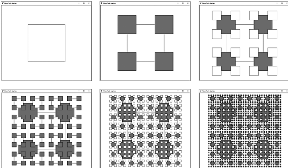
Рис. 13.8. Этапы создания фрактала «Четыре угла» слева направо и сверху вниз. Каждый рекурсивный вызов создает еще четыре квадрата по углам исходного, чередуя их цвета между белым и серым
