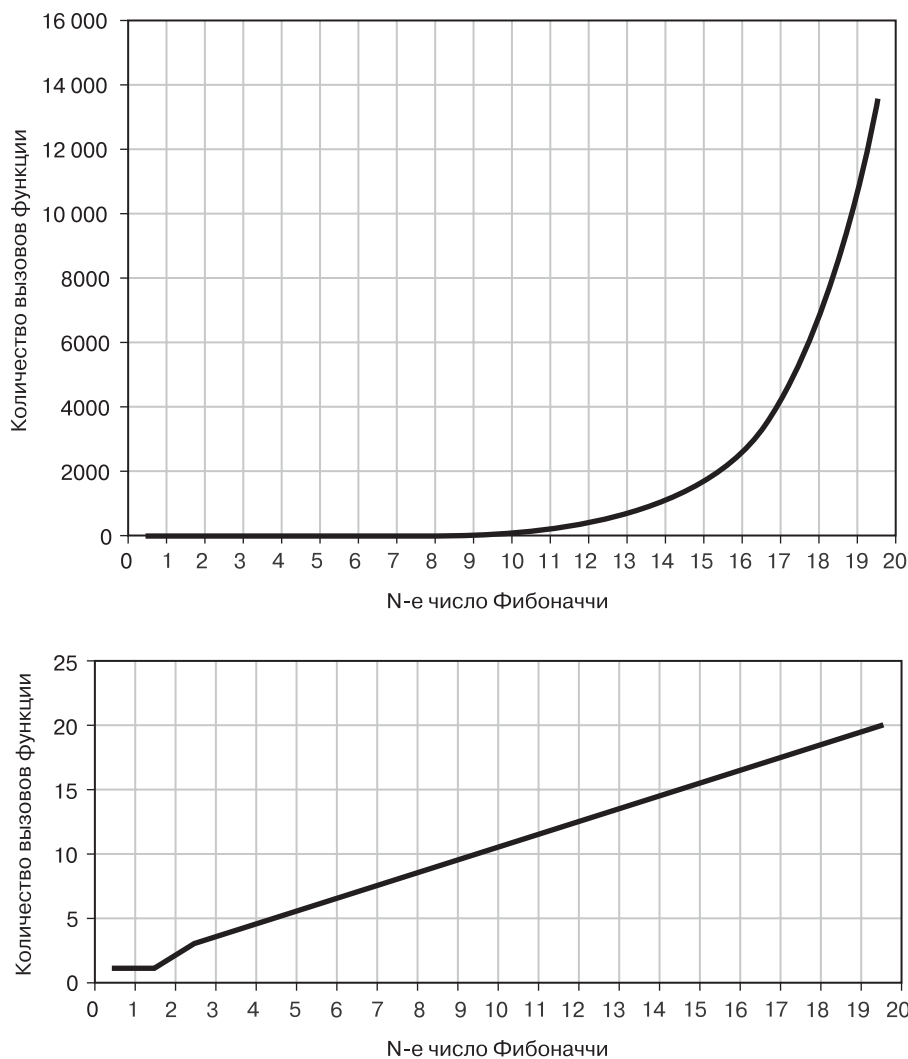
Рис. 7.2. Количество вызовов исходной функции fibonacci() растет очень резко (верхний график), чего нельзя сказать о ее мемоизированной версии (нижний график)
