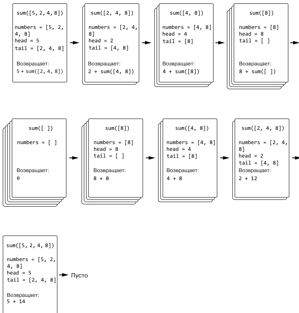
Рис. 3.1. Состояние стека вызовов для функции sum([5, 2, 4, 8])
