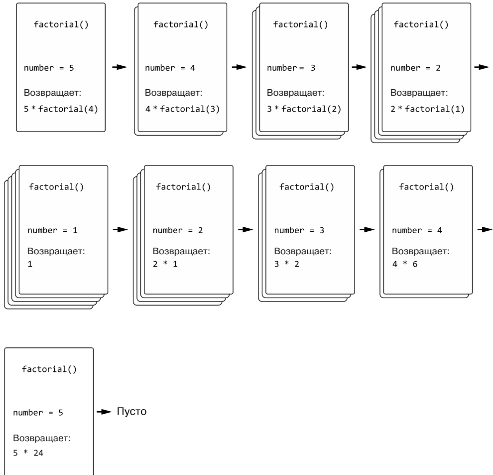
Рис. 2.1. Изменение состояния стека вызовов в результате многократного вызова рекурсивной функции factorial() и последующего возврата
