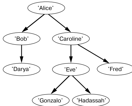
Рис. 4.4. Дерево, в котором хранятся имена, используемое в программах depthFirstSearch.py и depthFirstSearch.html
