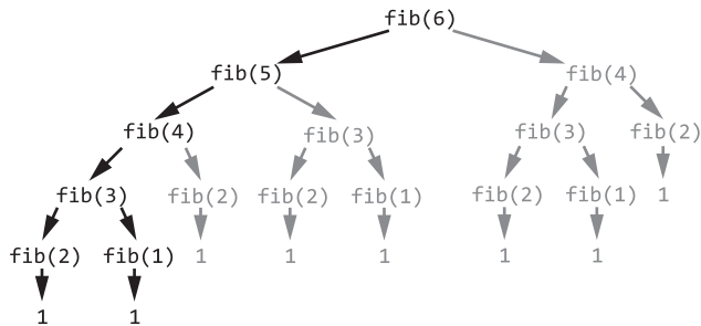
Рис. 2.3. Древовидная диаграмма рекурсивных вызовов функций, начиная с fibonacci(6) . Избыточные вызовы выделены серым цветом
