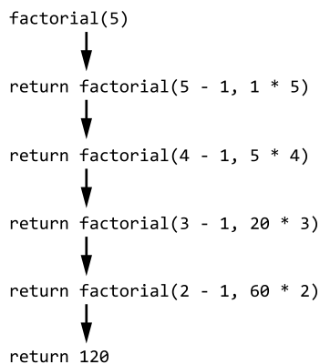
Рис. 8.1. Процесс преобразования factorial(5) в целое число 120
