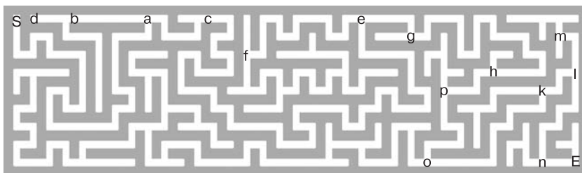
Рис. 4.5. Лабиринт, который проходит программа, описанная в этой главе. Развилки, обозначенные строчными буквами, соответствуют узлам графа на рис. 4.6
