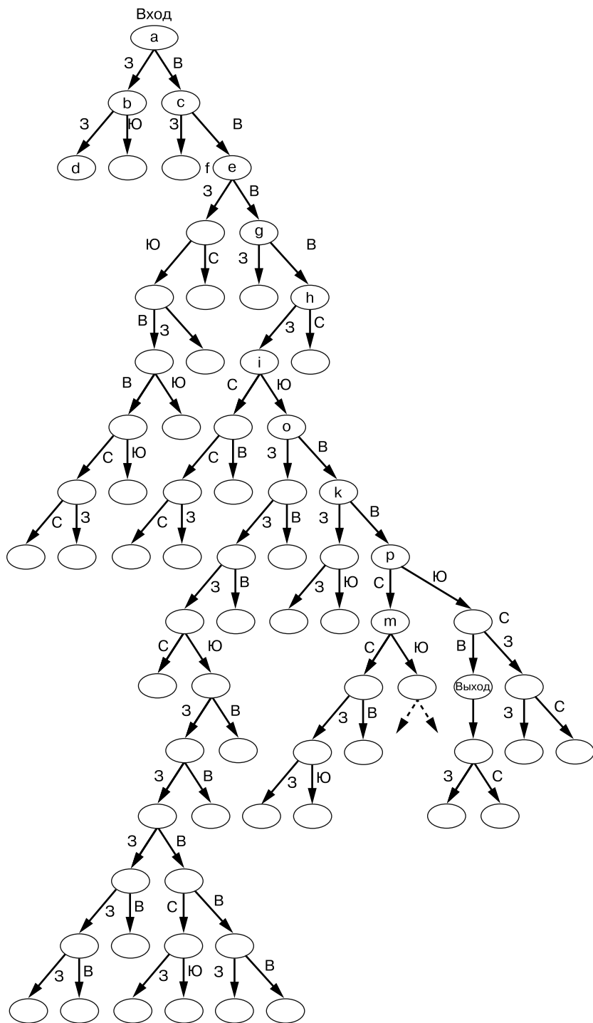
Рис. 4.6. В данном графе узлы обозначают развилки, а ребра — северное, южное, восточное или западное направления движения. Узлы, обозначенные строчными буквами, соответствуют развилкам на рис. 4.5
