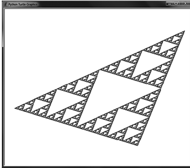
Рис. 9.6. Искаженный треугольник Серпинского
