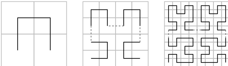
Рис. 9.17. Первые три шага создания кривой Гильберта
