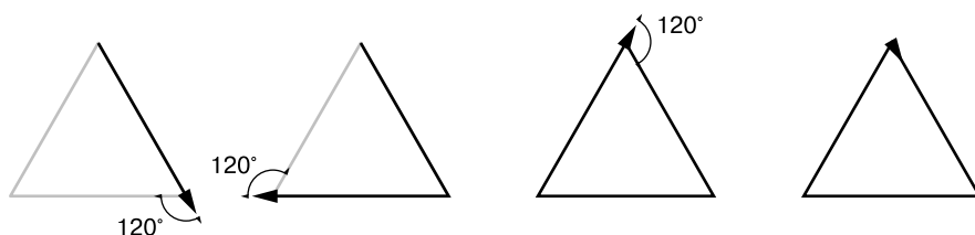
Рис. 13.7. Процесс рисования равностороннего треугольника предполагает трехкратное повторение перемещения с поворотом вправо на 120°
