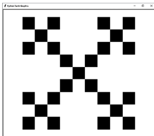
Рис. 9.20. Фрактал Вичека, нарисованный с использованием двух уровней рекурсии
