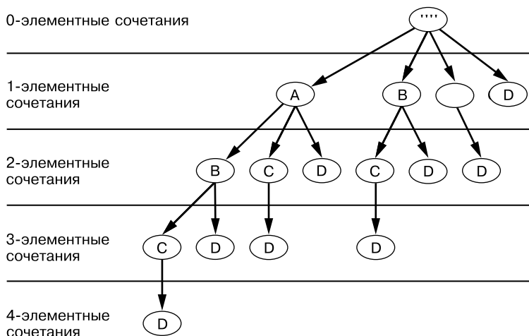
Рис. 6.4. Дерево, содержащее все возможные k -элементные сочетания (от 0 до 4) для множества \{A, B, C, D\}
