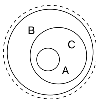
Рис. 6.1. Множество \{A, B, C\} , обведенное пунктирной линией, и его подмножества \{A, B, C\} , \{A, C\} и \{\} , обведенные сплошными линиями. Круги обозначают множества, а буквы — их элементы
