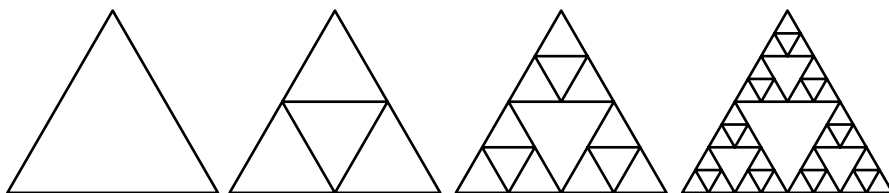
Рис. 9.3. Равносторонний треугольник (слева) и треугольники Серпинского, полученные путем рекурсивного добавления перевернутых треугольников
