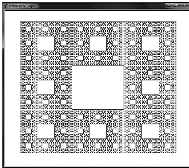
Рис. 9.9. Ковер Серпинского, образованный только контурами прямоугольников
