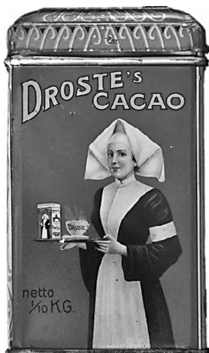
Рис. 14.1. Рекурсивная иллюстрация на банке какао Droste
