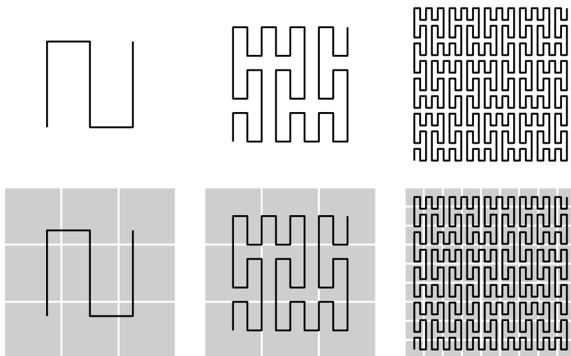
Рис. 9.21. Первые три итерации построения кривой Пеано (слева направо). В нижнем ряду показано разбиение заполняемой области по линиям сетки 3 \times 3 , в каждой из ячеек которой находится та или иная часть кривой
