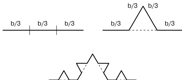
Рис. 9.14. Разделив линию на три равных отрезка (слева), добавьте равносторонний треугольник без основания (справа). Теперь мы имеем четыре отрезка длиной b/3 , к каждому из которых тоже можно добавить треугольник (внизу)
