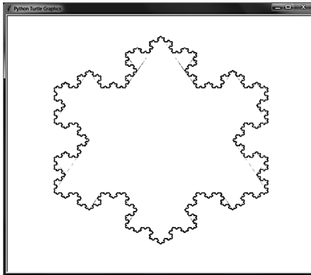
Рис. 9.16. Снежинка Коха. Часть внутренних линий остается из-за небольших ошибок округления
