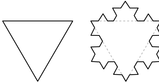
Рис. 9.15. Создание трех кривых Коха на трех сторонах равностороннего треугольника для формирования снежинки Коха
