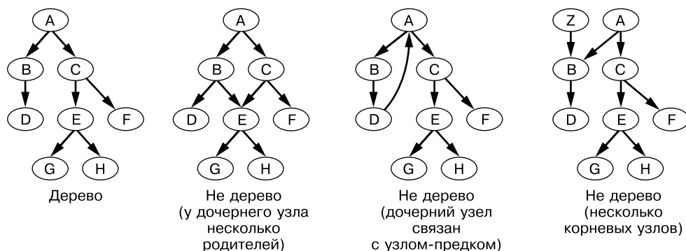
Рис. 4.1. Дерево (слева) и три структуры, не являющиеся деревьями
