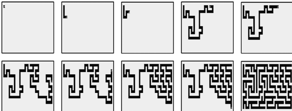
Рис. 11.1. Процесс создания лабиринта с помощью рекурсивного алгоритма поиска с возвратом
